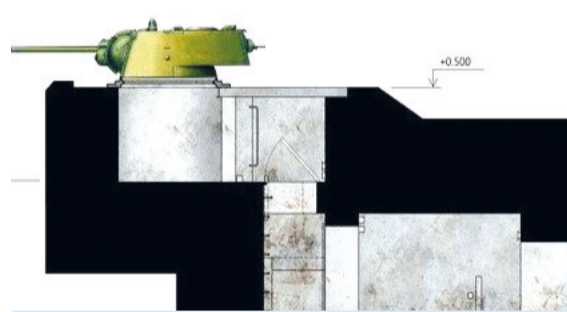
Схема устройства ДОТа с танковой башней
